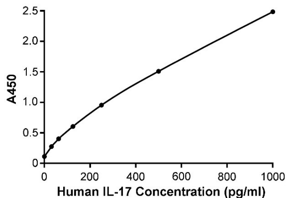
图3. Human IL-17 ELISA Kit的标准曲线。实测数据会因实验条件、检测仪器等的不同而存在差异，图中数据仅供参考。
